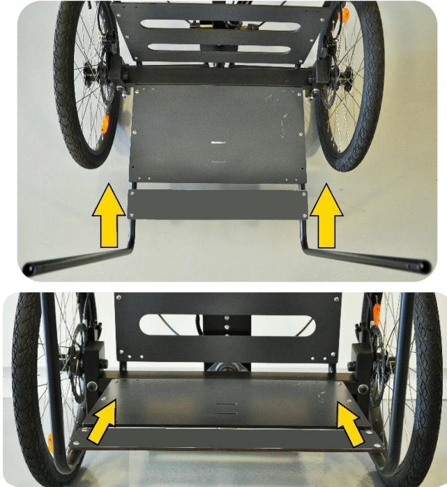
Figure 5 - Insertion des tubes bas dans l'assise
